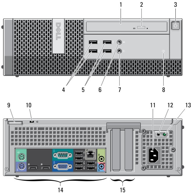
Angka 3. Tampilan Panel Belakang dari Small Form Factor
